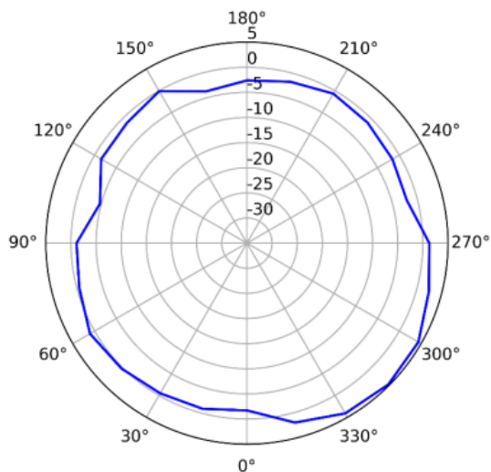
2.4GHz (Vertical)
