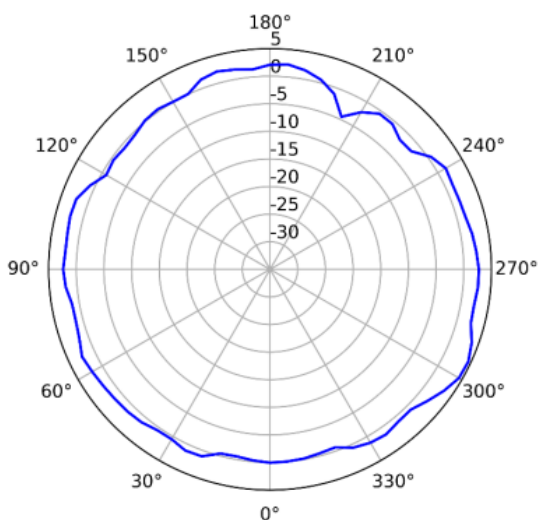
5GHz (Horizontal)
